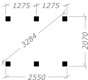
Fyrkantiga plintar (1:50)
