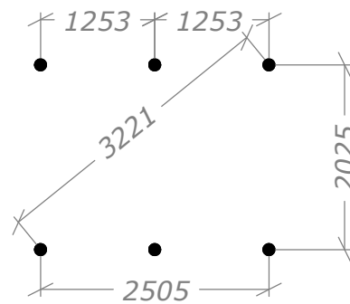
Runda plintar (1:50)
