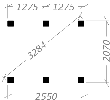
Fyrkantiga plintar (1:50)
