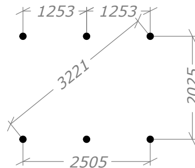
Runda plintar (1:50)
