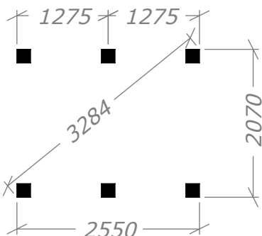
Fyrkantiga plintar (1:50)
