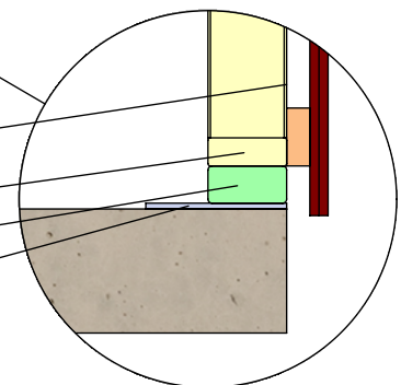
DETAIL E 1 : 10
