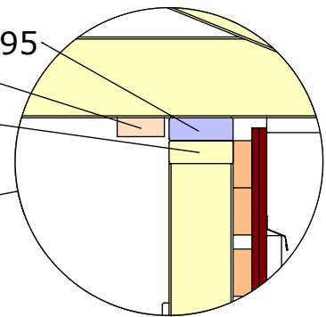
DETAIL D 1 : 10
